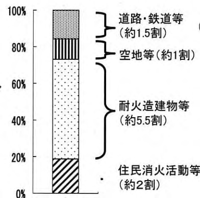
図：兵庫県神戸市水笠西公園周辺火災の延焼動態図と焼け止まり要因 (出典：平成7年兵庫県南部地震被害調査最終報告書)
