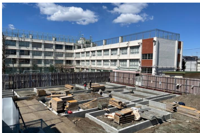
▲基礎工事の様子
