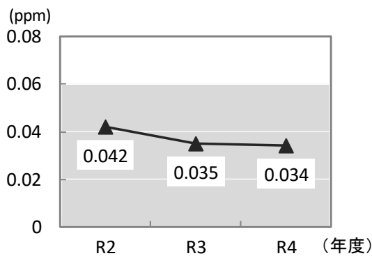
＜二酸化窒素濃度の推移＞
