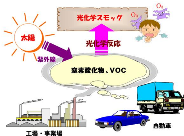
<光化学スモッグ発生のメカニズム> (都ホームページより引用)
