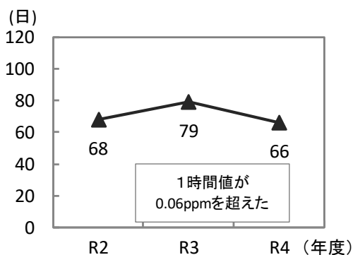
＜光化学オキシダント濃度が環境基準値を超えた日数の推移＞
