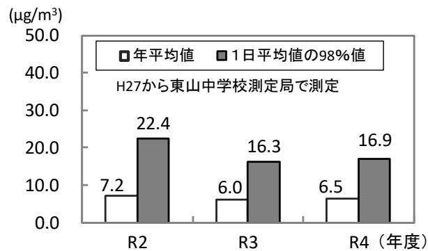
＜微小粒子状物質（PM2.5）の測定結果＞
