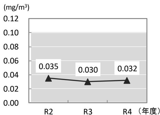
＜浮遊粒子状物質含有量の推移＞
