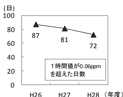
＜光化学オキシダント濃度が環境基準値を超えた日数の推移＞
