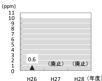
＜一酸化炭素濃度の推移＞
