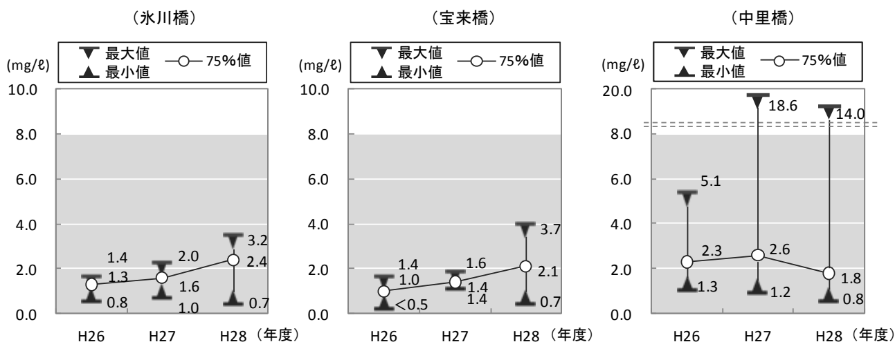
＜目黒川のBOD濃度の推移＞
