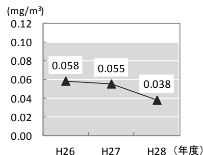
＜浮遊粒子状物質含有量の推移＞
