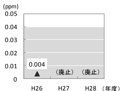
＜二酸化硫黄濃度の推移＞
