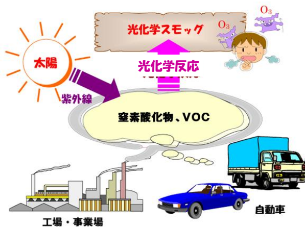
＜光化学スモッグ発生メカニズム＞ （都ホームページより引用）
