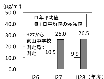
＜微小粒子状物質（PM2.5）の測定結果＞
