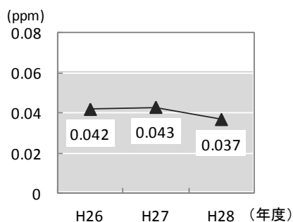
＜二酸化窒素濃度の推移＞
