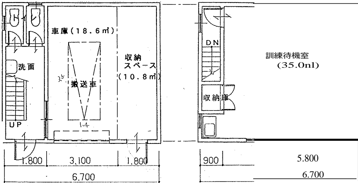
2 階平面図
