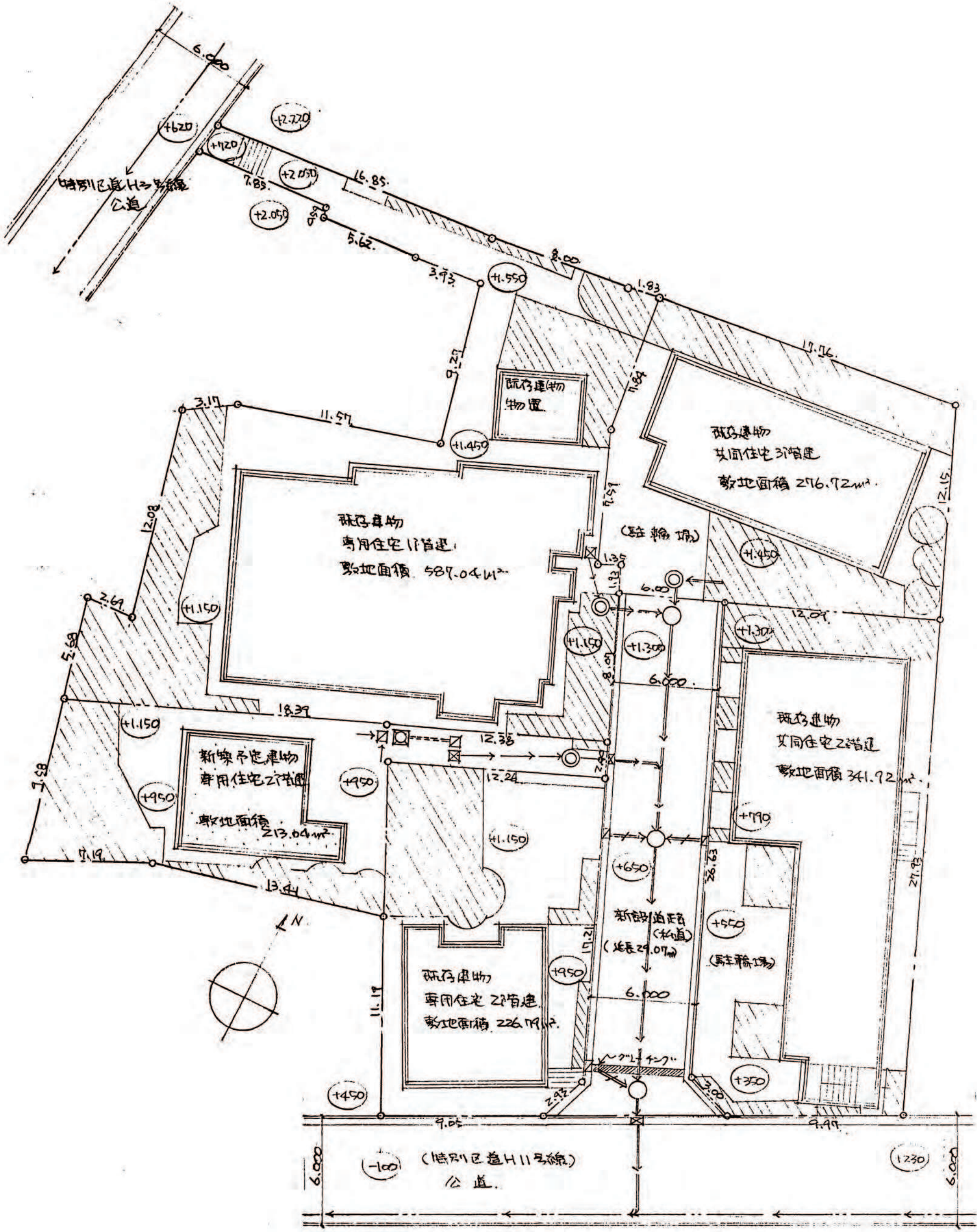
土地利用計画図 1:200
