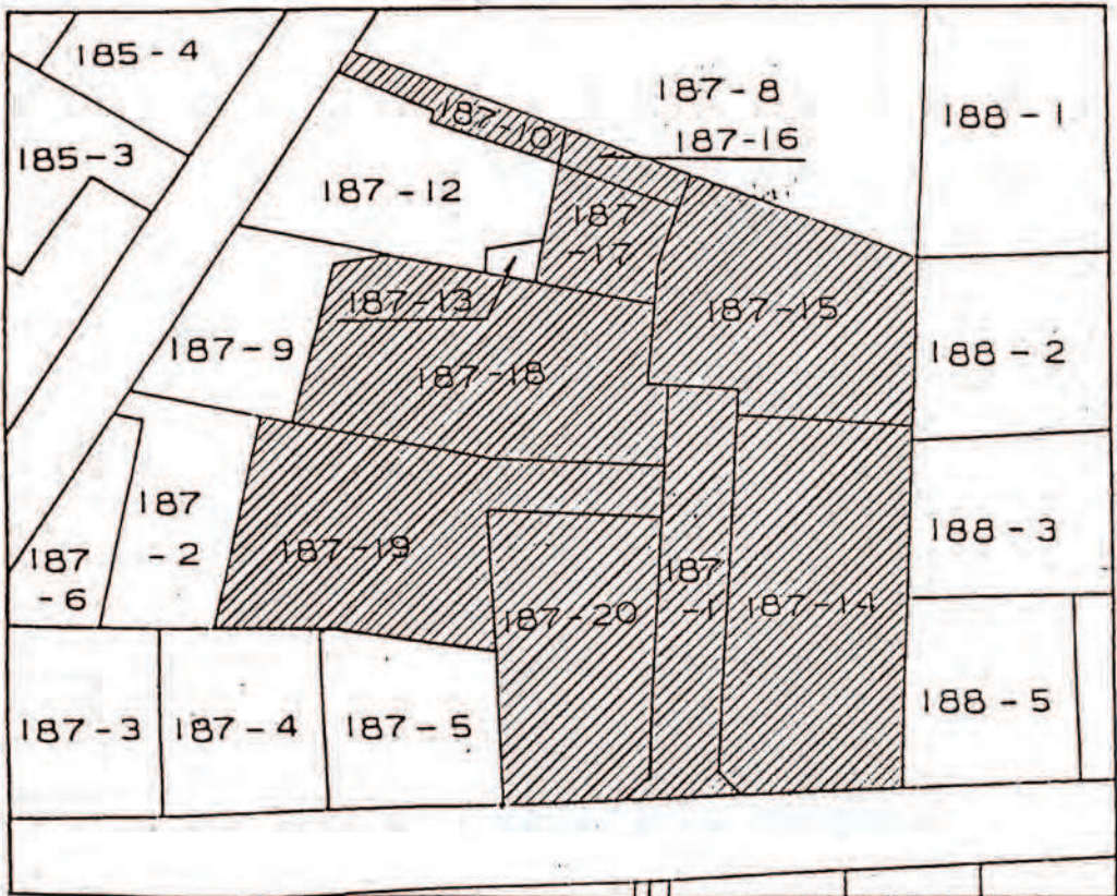
公図写 1:600
