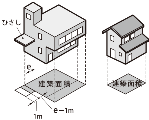
図 1 建 蔽 率
