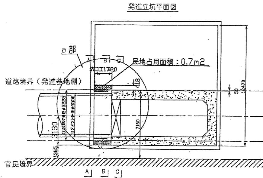
管理境界占用範囲図 縮尺1/200
