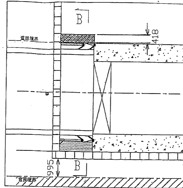
a部詳細図(B-B) 縮尺1/100
