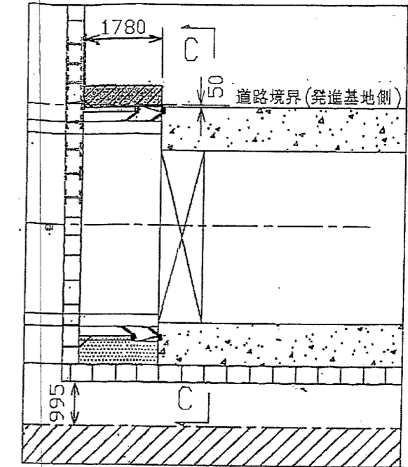
a部詳細図(C-C) 縮尺1/100
