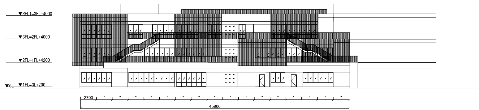
北側立面図
