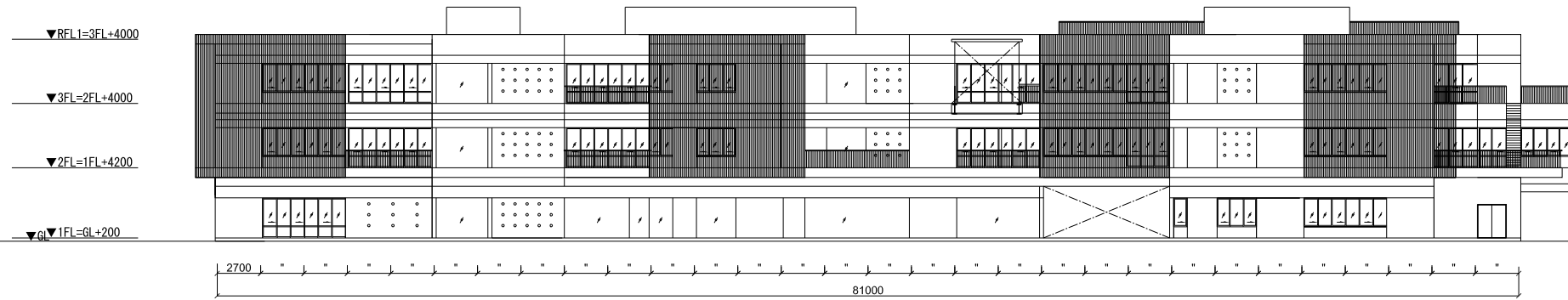
東側立面図
