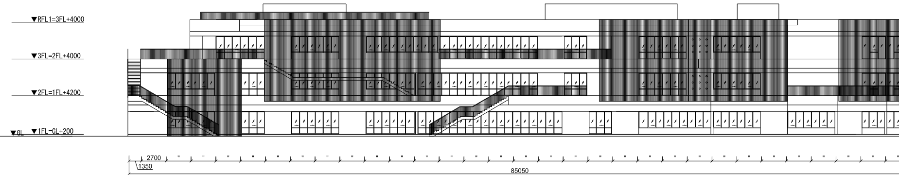
西側立面図
