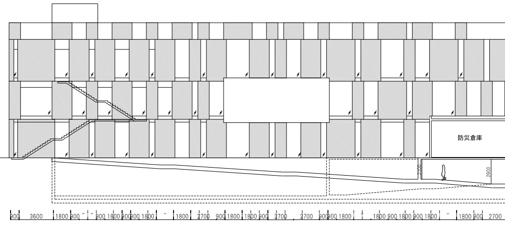
東側立面図
