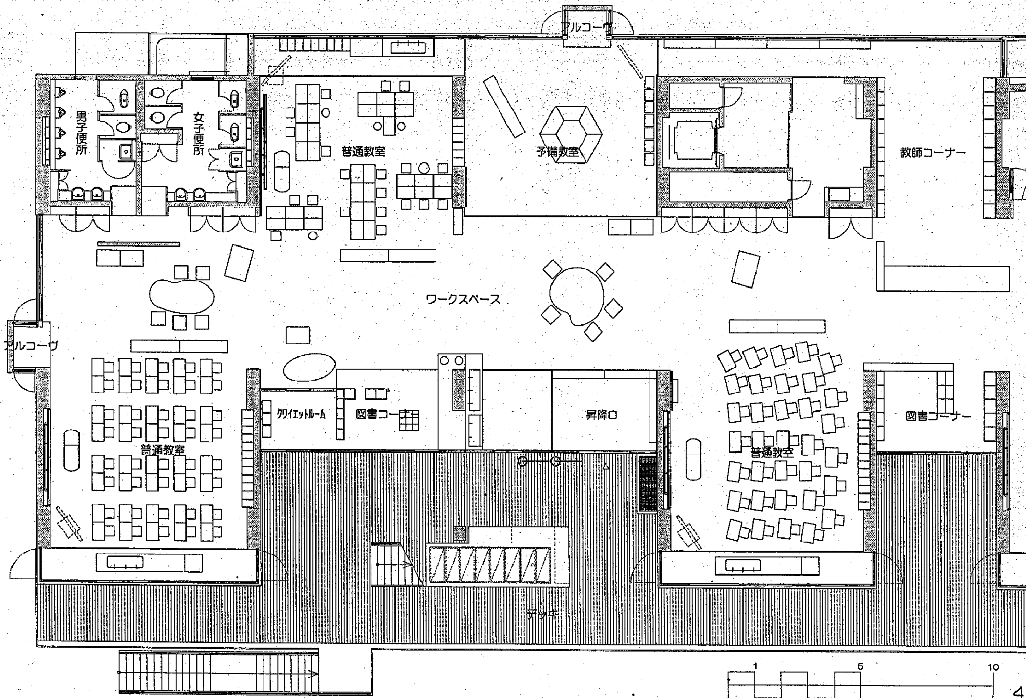
[教室平面詳細図]
