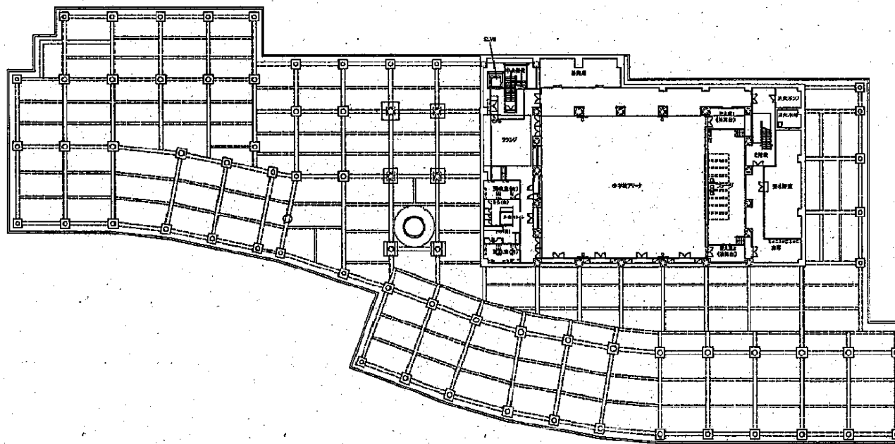
地下1階平面圖
